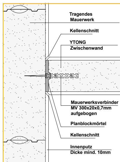
Starrer Wandanschluss
