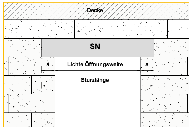
Einbau SN
