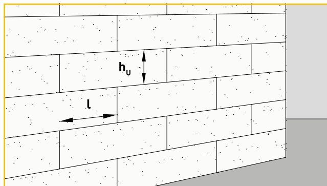
Überbindemaß (l) \geq 0,4 h_u
