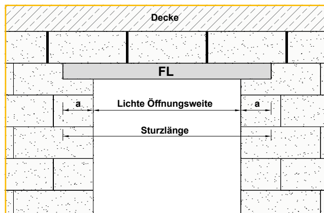
Einbau FL
