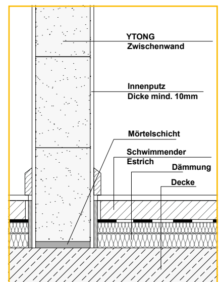
Starrer Fußpunkt
