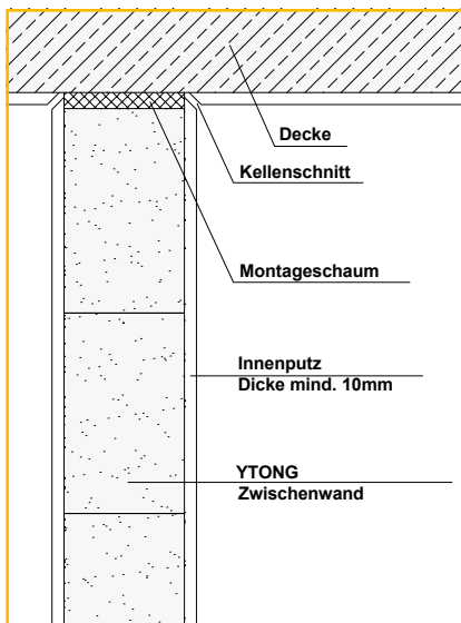
Gleitender Deckenanschluss
