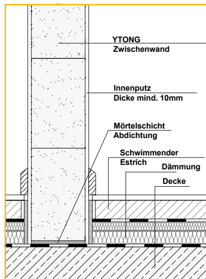
Gleitender Fußpunkt
