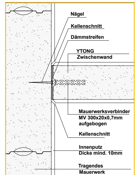
Gleitender Wandanschluss
